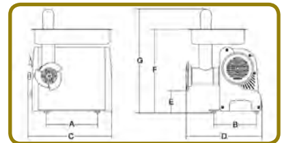
ESQUEMA DIMENSIONES (mm)
