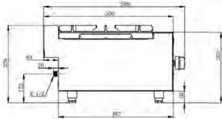
ESQUEMA LATERAL MODELOS CHP-112/224/336
