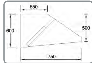
ESQUEMA DIMENSIONES
