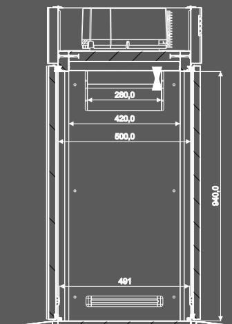
RIC1PTH Pasante/Pass-thru/Traversante
